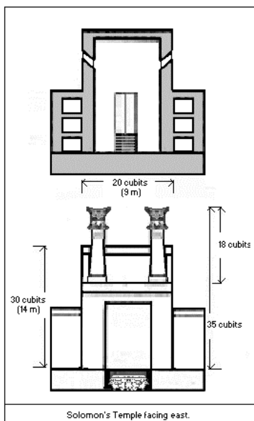
Ricostruzioni ipotetiche del Tempio di Salomone.
