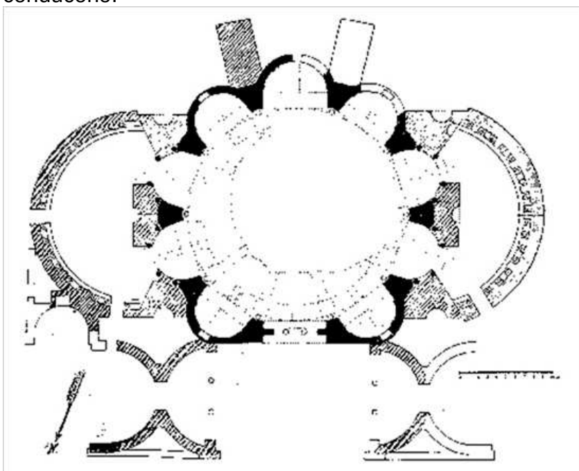
Pianta di Minerva Medica
